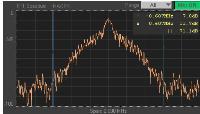
Fig. 45: FFT spectrum display
